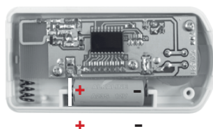
Obr. 6 Polarita batérie
